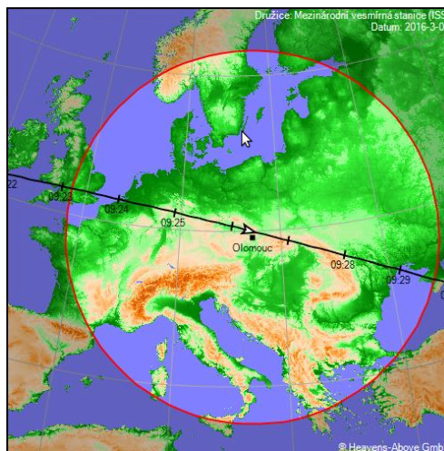
Obr. 4: Přelet ISS nad Evropou 8. 3. 2016 dopoledne. Kružnice vymezuje oblast, nad níž by ISS byla z Olomouce vidět výš než 10° nad obzorem. Zdroj: Heavens-Above, http://www.heavens-above.com
